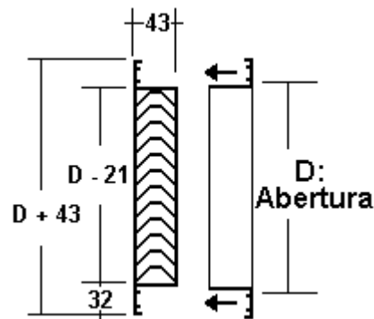
AL 251 NV (Marco sin Montar)
